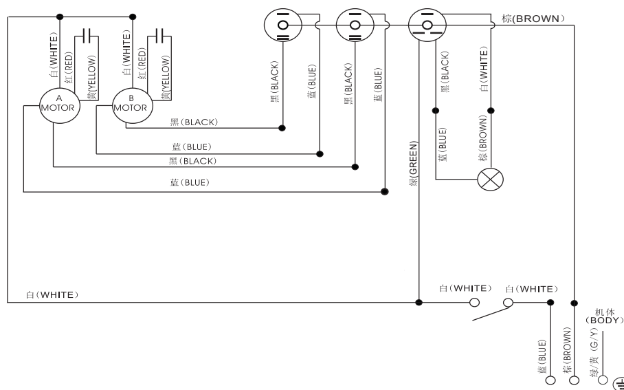
雙摩打抽油煙機線路圖
